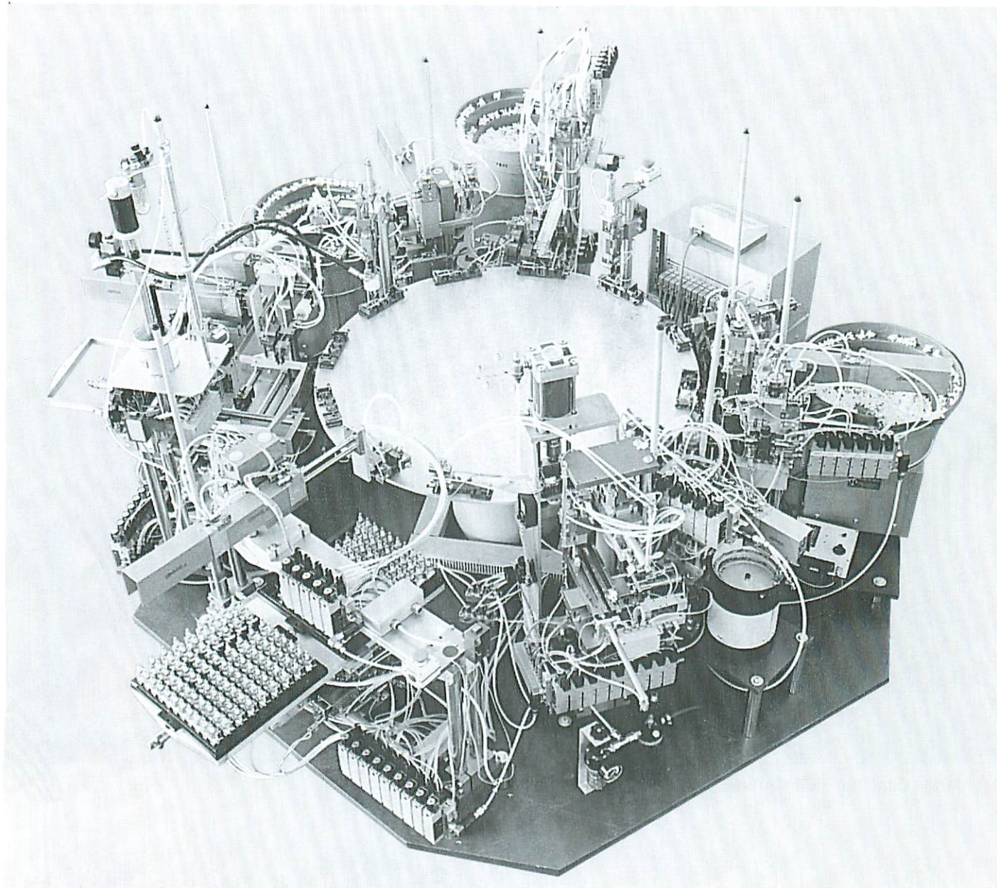
Montageanlage zum Montieren von Baugruppen für Radios
